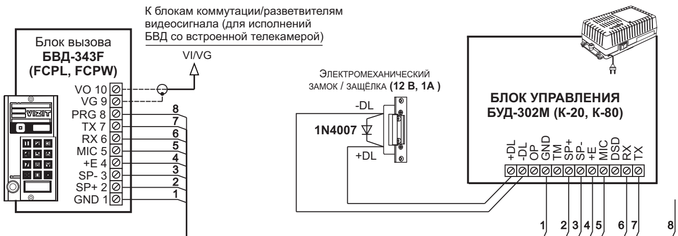
Рисунок 8 - Схема соединений блока вызова БВД-343F(FCPL, FCPW) с блоком управления БУД-302М (К-20, К-80) и электромеханическим замком / защёлкой
